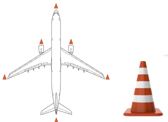
Przykład rozmieszczenia pachołków bezpieczeństwa oraz przykładowy pachołek
