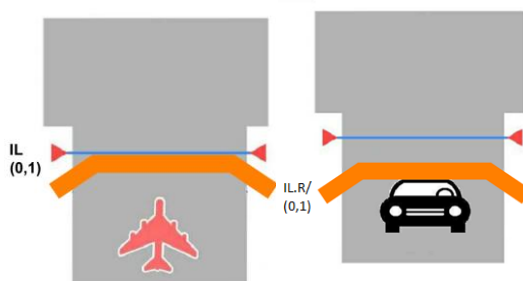
Układ pojedynczych pętli na drogach kołowania i drogach ruchu kołowego.
