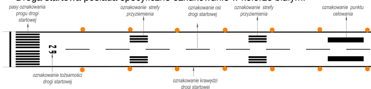
Oznakowanie drogi startowej.
