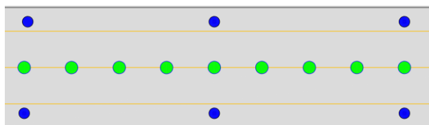
Oświetlenie dróg kołowania. Krawędzie koloru niebieskiego i osi – zielone.
