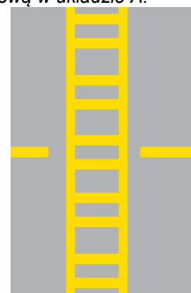
Oznakowanie poziome miejsca oczekiwania przed drogą startową w układzie B.
